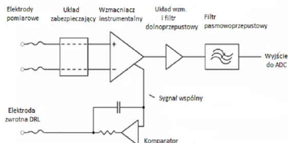
Rysunek 36: Schemat ideowy wzmacniacza biologicznego [15].
