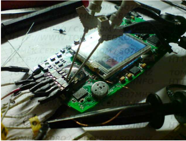
Rysunek 42: Trwają prace nad stworzeniem otwartego narzędzia do pracy z układami wyposażonymi w magistralę SWD.
