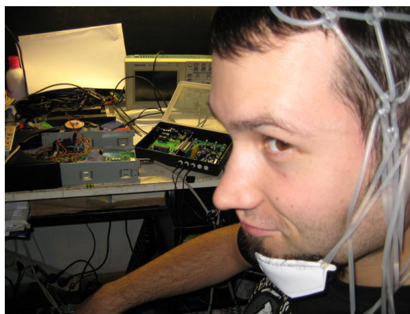
Rysunek 48: Badanie EEG wykonywane za pomocą OpenEEG oraz porównawczo naszego autorskiego urządzenia.
